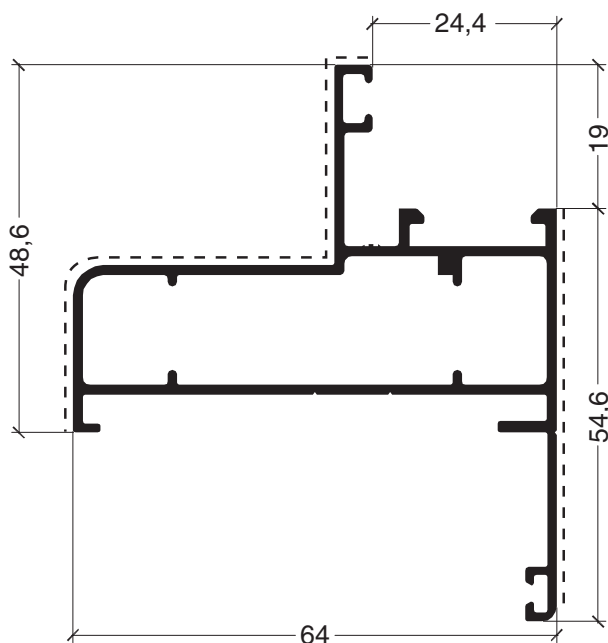
ADR 1513 Marco 64 mm con tapajuntas 0,952 kg/m
