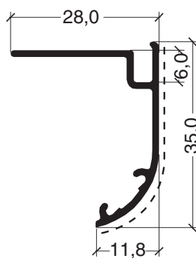
ADR 1662 Tapajuntas 0,277 kg/m
