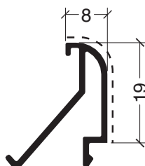
ADR 1174 Contravidrio curvo 16 mm 0,220 kg/m
