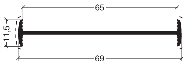
ADR 1165 Perfil de unión 64 mm 0,364 kg/m
