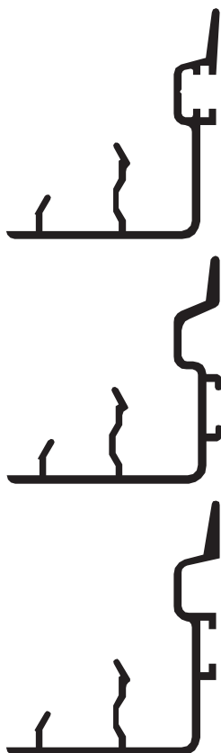
Calado pasaje de guías
