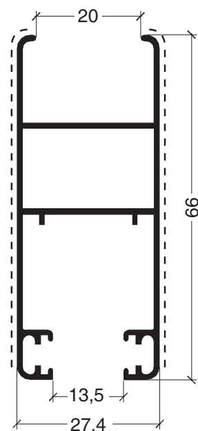
ADR 425 Hoja corte a 45° para DVH 0,697 kg/m
