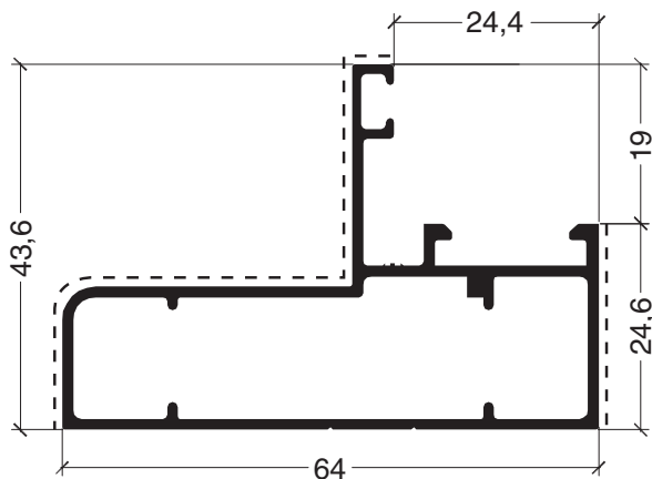
ADR 1160 Marco 64 mm 0,766 kg/m
