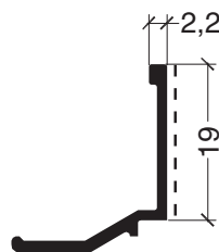
ADR 1178 Contravidrio para DVH 0,147 kg/m
