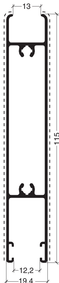
ADR 292 Zócalo alto /travesaño 1,081 kg/m
