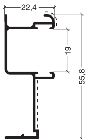
ADR 294 Guía cortina común 0,414 kg/m
