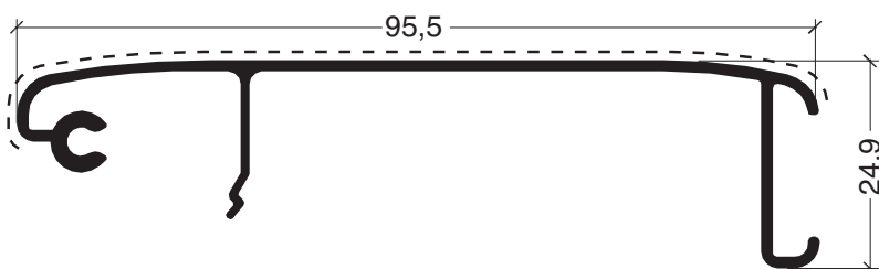
ADR 1653 Tapacinta 0,628 kg/m
