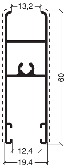
ADR 52A Zócalo/Cabezal hoja corte a 90° 0,593 kg/m
