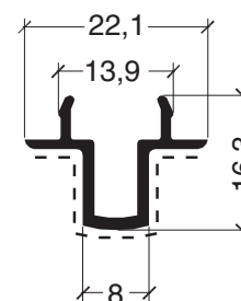
ADR 1651 Encuentro central 4 hojas 0,180 kg/m
