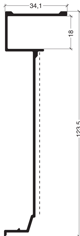
ADR 1381 Guía cortina barrio 0,753 kg/m
