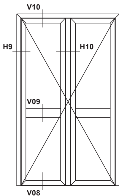
Puerta de rebatir de 2 hojas
