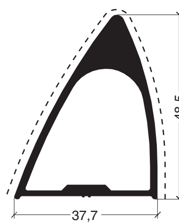
ADR 1515 Refuerzo de parante central 1,100kg/m
