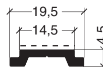
ADR 922 Pletina 0,139 kg/m
