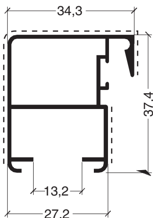
ADR 54 Parante central hoja corte a 90° 0,676 kg/m
