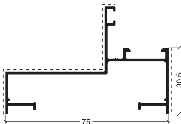
ADR 1176 Marco 75 mm 0,700 kg/m
