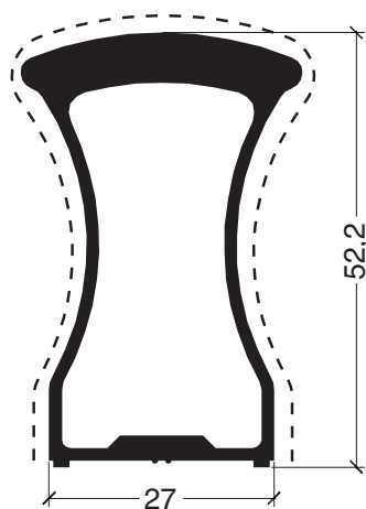
ADR 400 Refuerzo de parante central 1,042 kg/m
